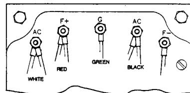
SCR MODULE
