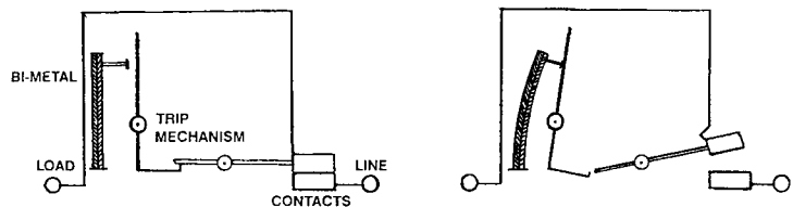
THERMAL TRIP
